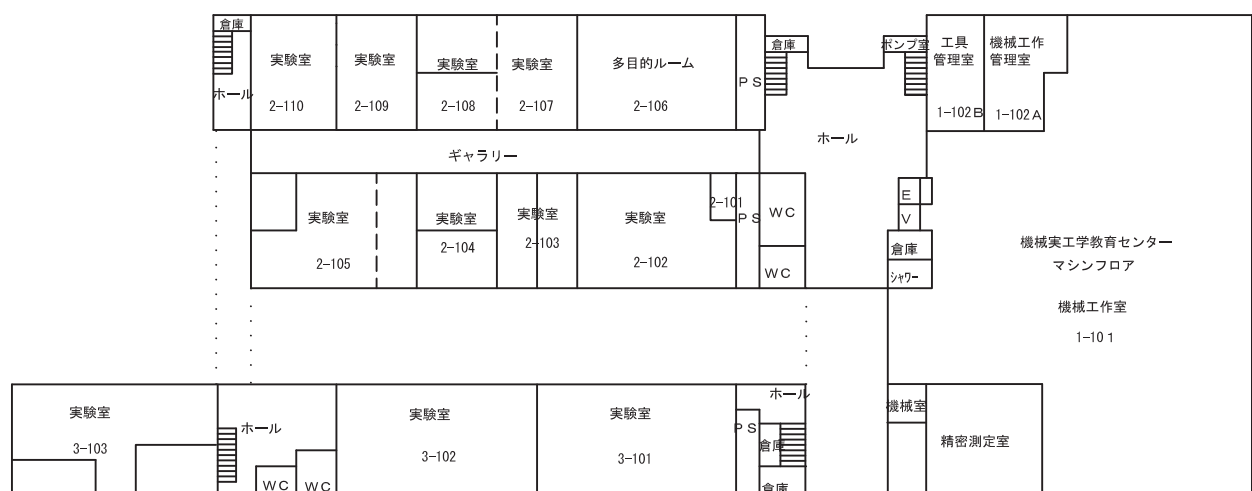
1階平面図
