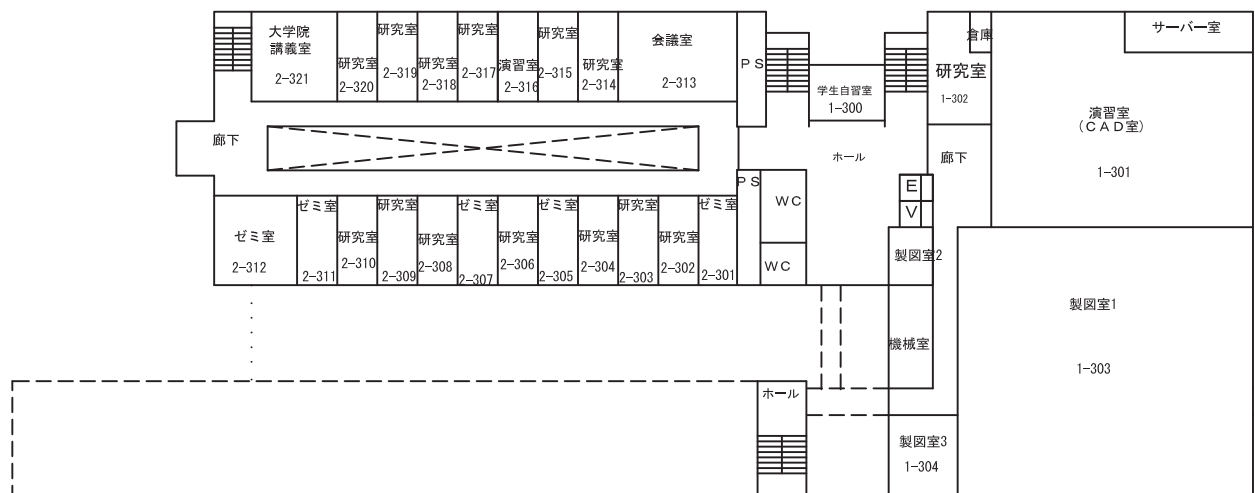
3 階平面図
