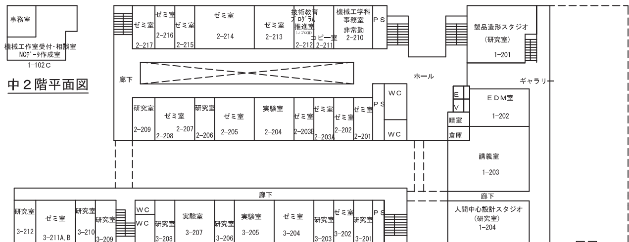
2階平面図
